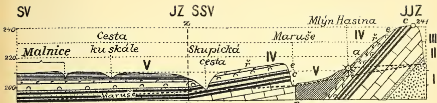
Obr. 34. Průřez pravé straně Maruše mezi Lipencem a Malnicemi.
