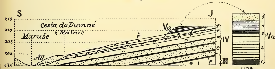
Obr. 37. Průřez dle Skupické cesty.
