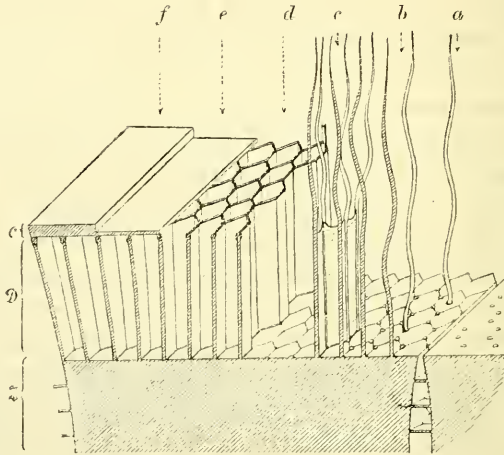
Schematische Darstellung der Structure der Deckplatte. Links die fertige Deckplatte mit einer Cuticula (e, f.), rechts flimmernde Cilien (b), in der Mitte hypothetische Uebergangsstadien (c) d) — Deckplatte ohne Cuticula, Z—Zelle, D—Deckplatte, C—Cuticula.
