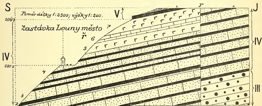
Obr.32. Profil nad zastávkou „Louny - město“
