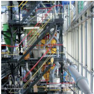
Centrale thermique à lit fluidisé
