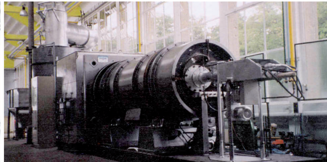
Unité de valorisation thermique de déchets
