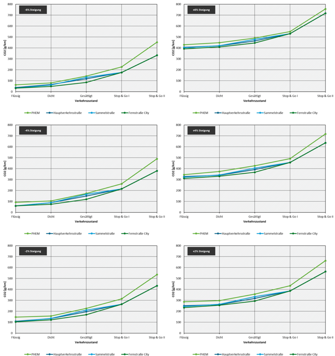
Abbildung 42: CO 2 -Emissionen für 5 % Schwerverkehr und variiertes Steigung
