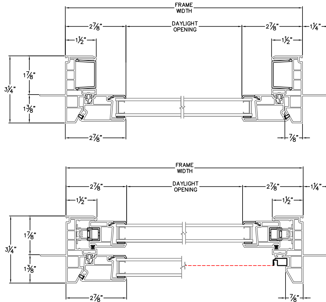
JAMBS
