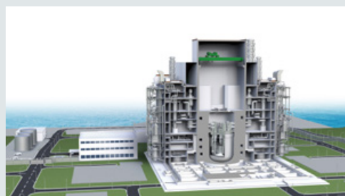
ナトリウム冷却タンク型高速炉 (経済産業省委託事業研究成果を含む)
