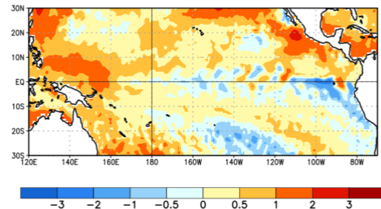
Rajah 2: Purata anomali suhu permukaan laut ( ^{\circ}\text{C} ) untuk minggu berpusat pada 04 September 2024
