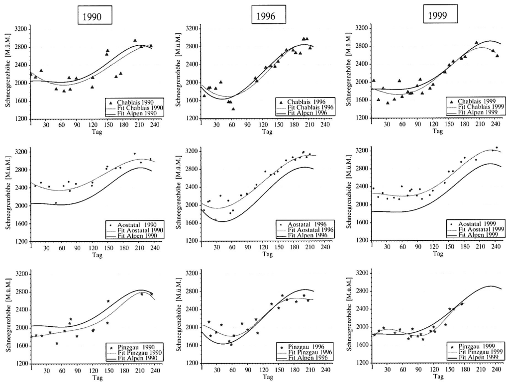
Fig. 8: The snow line evolution in the regions «Chablais» (top row), Aosta Valley (middle row) and «Pinzgau» (bottom row) indicate differences in climatic behavior in the Alps. Worth mentioning is the higher snow line elevation in the inner alpine regions. Day 1 denotes the first of January. Die Schneegrenz-Signaturen der drei Regionen «Chablais» (oben), Aostatal (Mitte) und Pinzgau (unten) dokumentieren unterschiedliche Klimaregime in den alpinen Regionen. Markant ist die permanent höher liegende Schneegrenze in inneralpinen Tälern. Tag 1 entspricht jeweils dem 1. Januar. L'évolution de la limite neigeuse des trois régions «Chablais» (en haut), «Val d'Aoste» (au milieu) et «Pinzgau» (en bas) témoigne des régimes climatiques différenciés dans les régions alpines. Il convient de souligner le fait que dans les vallées intraalpines la limite neigeuse permanente supérieure est située à une altitude plus élevée qu'ailleurs. Le premier jour correspond au 1. janvier.
