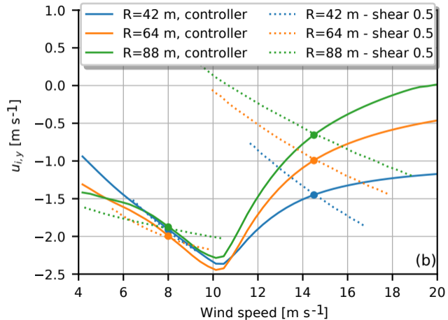
Grid BEM
