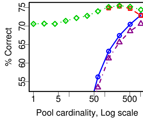
(d) 1024 codewords
