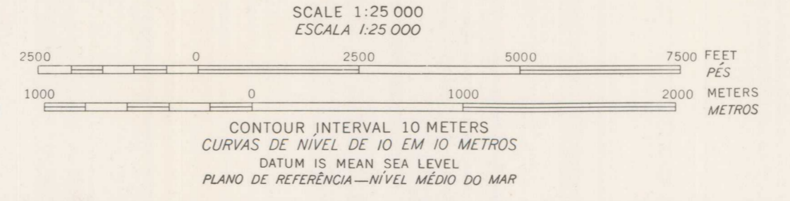
GEOLOGIC SECTIONS OF THE SÃO BARTOLOMEU, ANTÔNIO PEREIRA, OURO PRÊTO, SANTA RITA DO OURO PRÊTO MARIANA, AND RIO DAS BANDEIRAS QUADRANGLES, MINAS GERAIS, BRAZIL SEÇÕES GEOLÓGICAS DAS QUADRÍCULAS DE SÃO BARTOLOMEU, ANTÔNIO PEREIRA, OURO PRÊTO, SANTA RITA DO OURO PRÊTO MARIANA E RIO DAS BANDEIRAS, MINAS GERAIS, BRASIL
