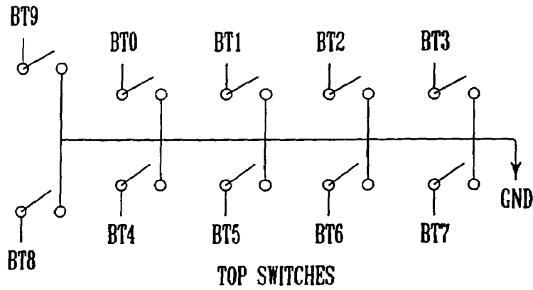
TOP SWITCHES FIG. 9A-3
