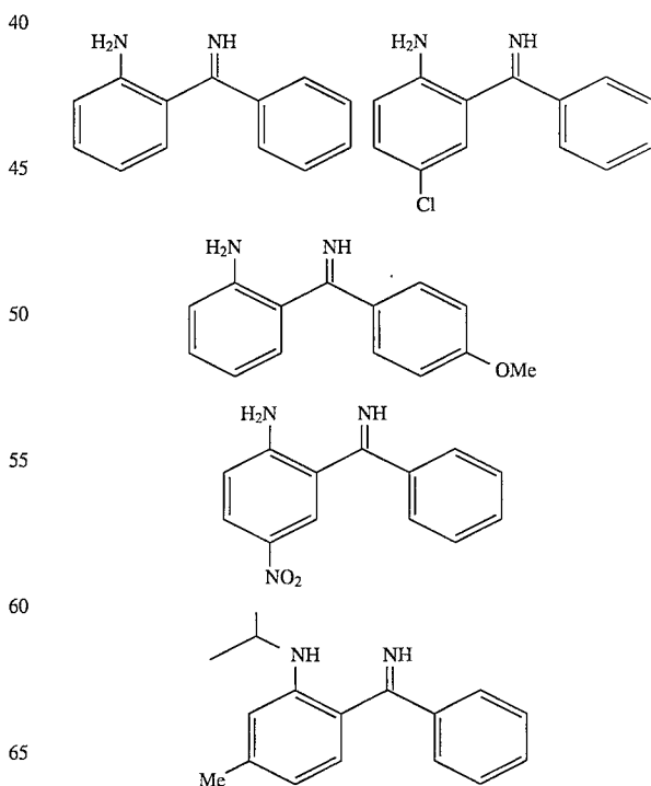
Imines:
