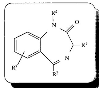
Imines:
