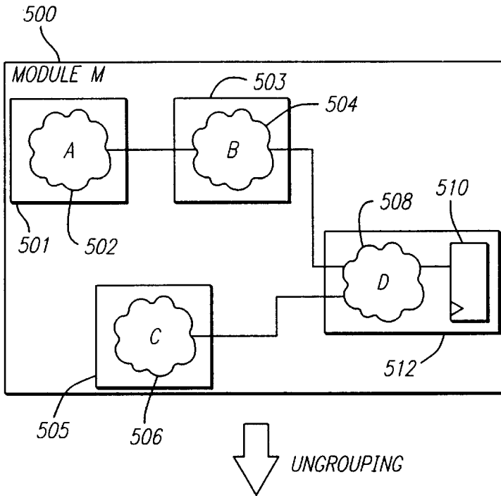
FIG. 22 HIERARCHY UNGROUPING
