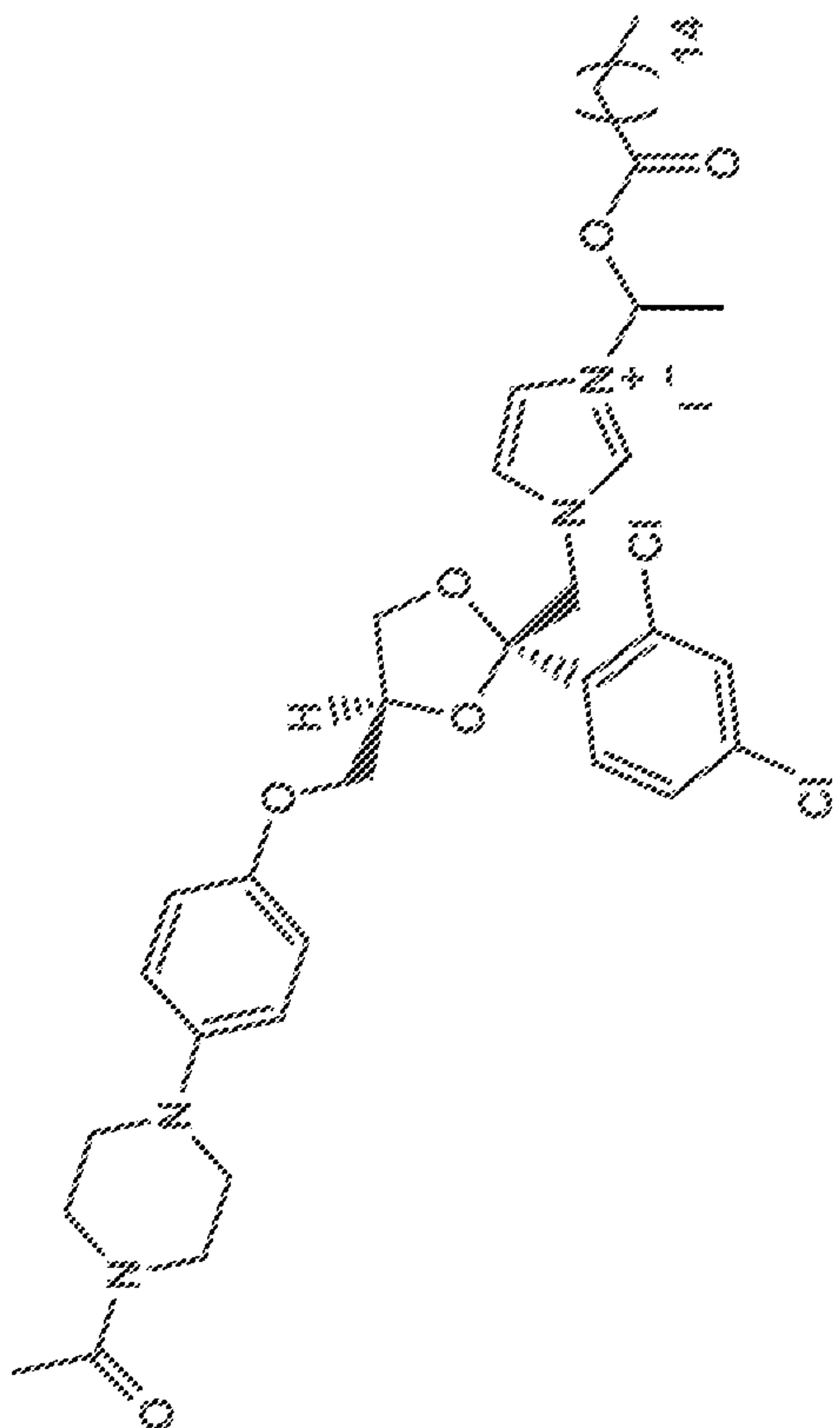
Ketoconazole-1-ethylenepalmitate conjugate
