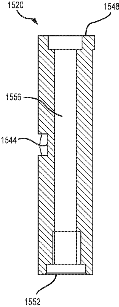
SECTION F-F FIG. 15F
