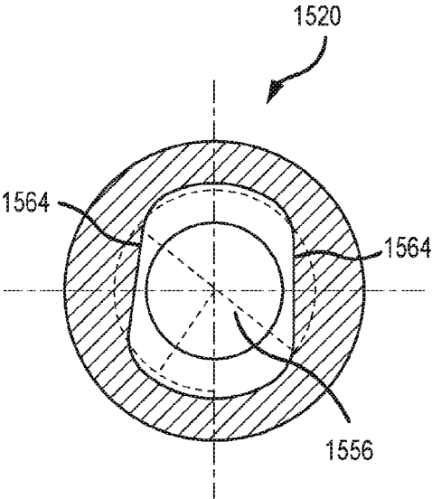
SECTION G-G FIG. 15G
