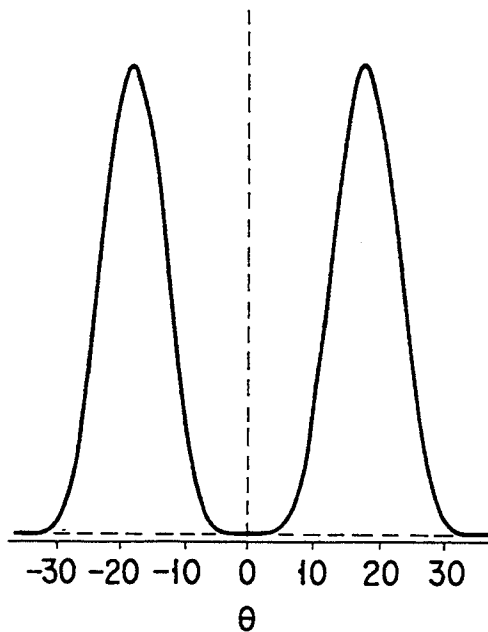
LP31 MODE
