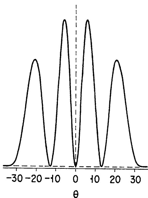
LP12 MODE
