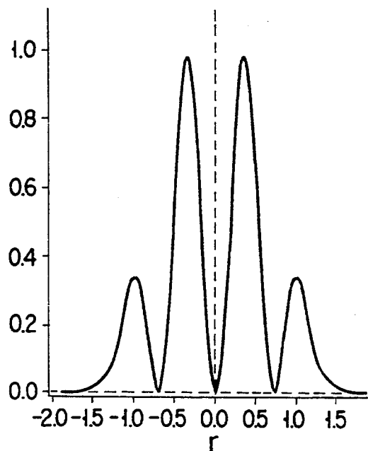
LP12 MODE
