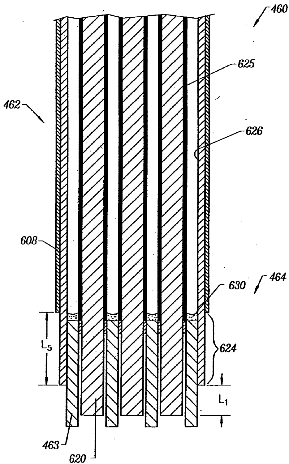
FIG. 17A
