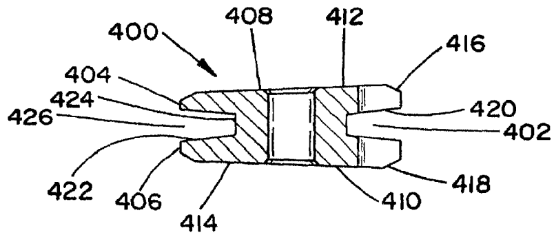
Section A-A FIG. 4c
