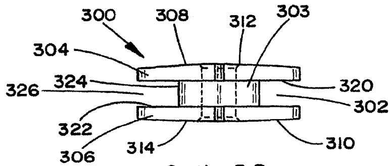
Section B-B FIG. 3b
