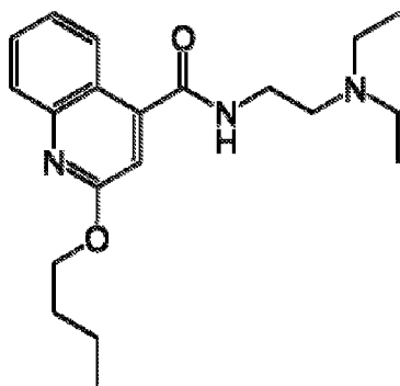
CINCHOCAINE
