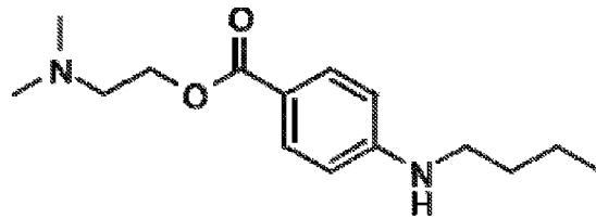
TETRACAINE
