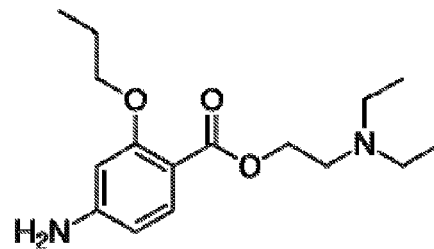
PROPOXYCAINE
