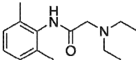
LIDOCAINE
