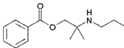
MEPRYLCAINE
