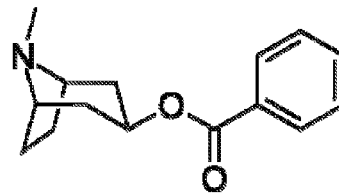
TROPACOCAINE
