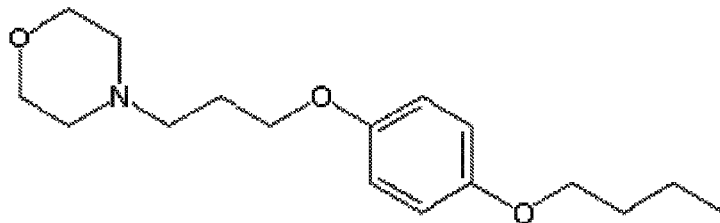
PRAMOCAINE
