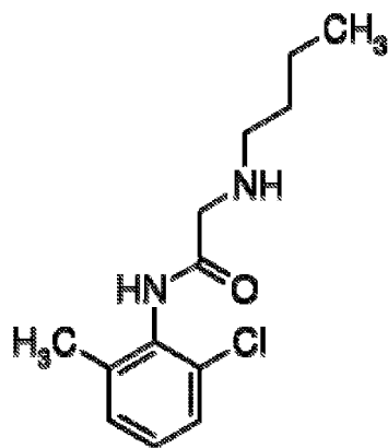
BUTANILCAINE
