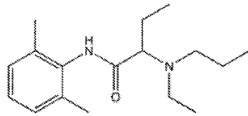
ETIDOCAINE
