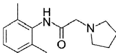
PYRROCAINE
