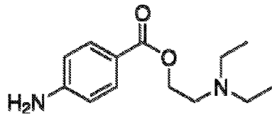
PROCAINE
