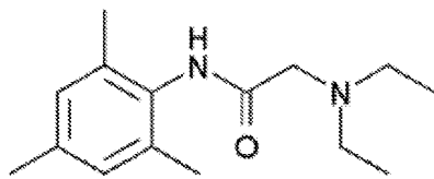
TRIMECAINE
