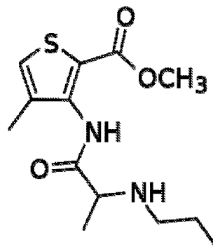
ARTICAINE
