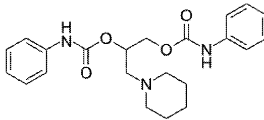
DIPERODON
