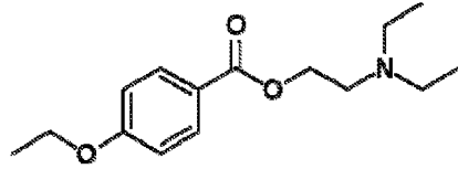
PARAETHOXYCAINE
