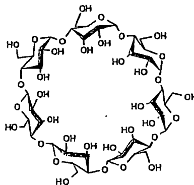
\beta -CD
