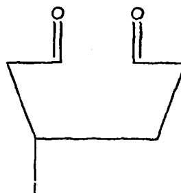
VIIc
