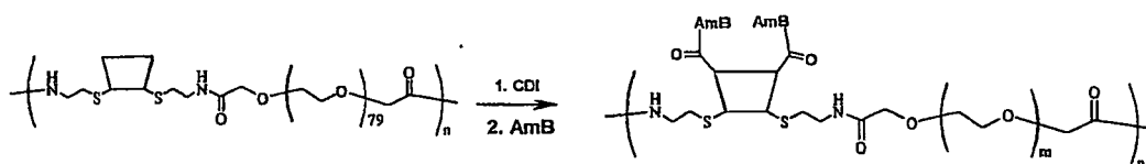
Scheme LII
