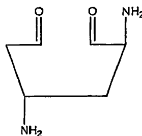
VIIIc
