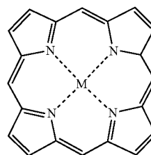
porphyrin
