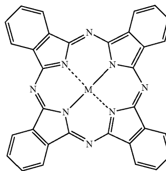
phthalocyanine M(Pc)
