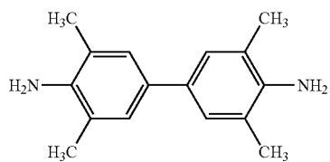
TMB
