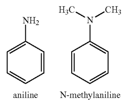
Formulae (D3): amine type donor
