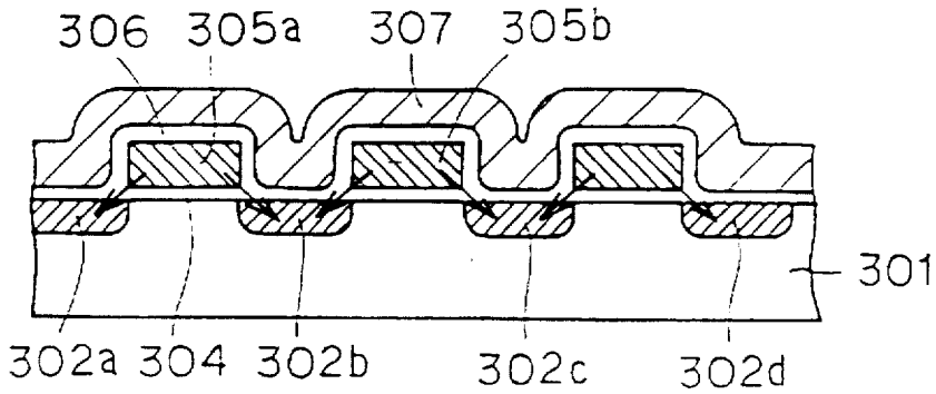
FIG. 158 PRIOR ART
