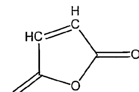
Maleic Anhydride
