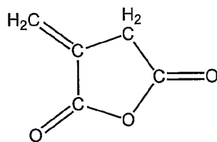
Itaconic Anhydride
