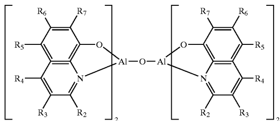
[Chem 3]
