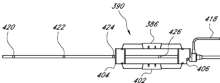
FIG. 29C
