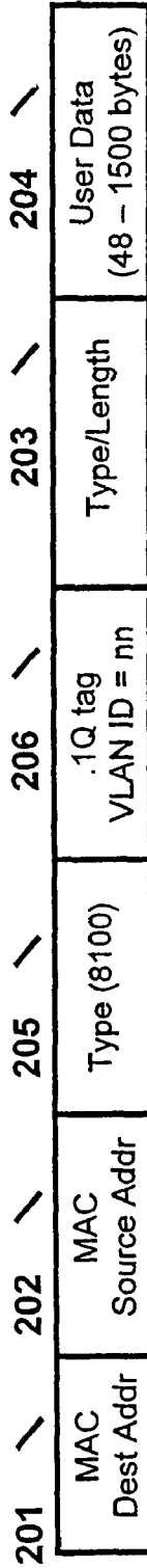
Fig. 2b - 802.1Q Tagging Format Packet (1514 + 4 bytes)
