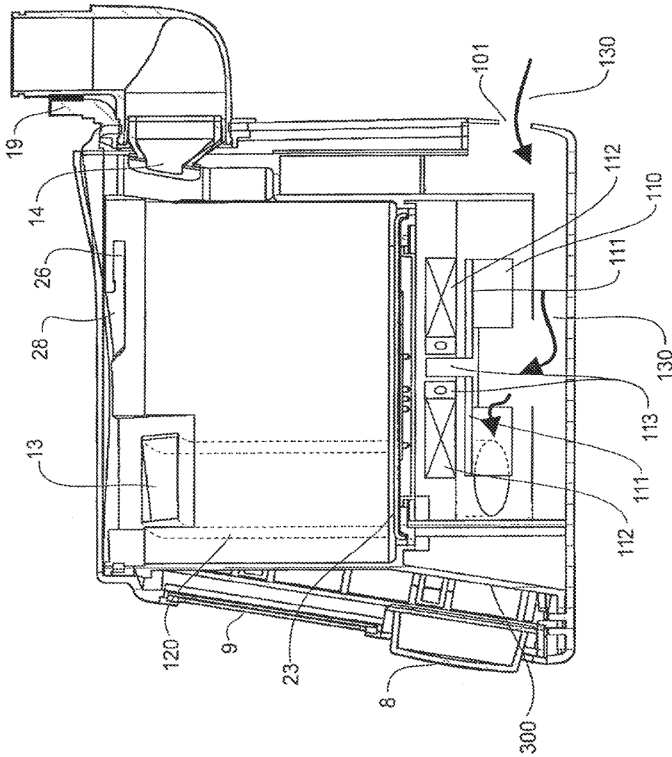
SECTION DD
