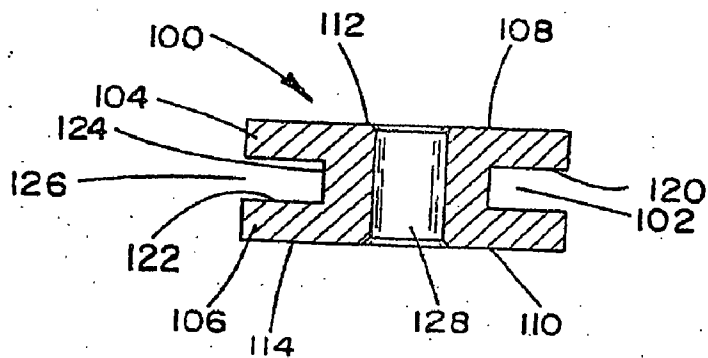
Section A-A FIG. 1c
