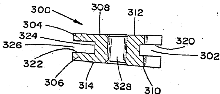
Section A-A FIG. 3c
