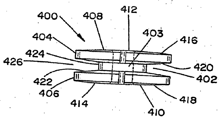
Section B-B FIG. 4b
