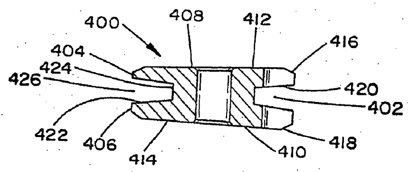
Section A-A FIG. 4c
