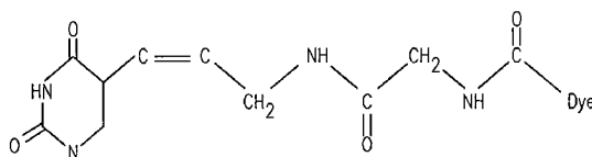
Diglycyl linker
