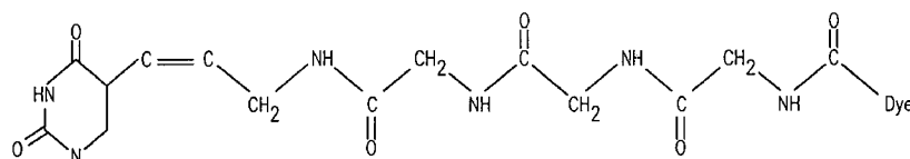
Tetraglycyl linker
