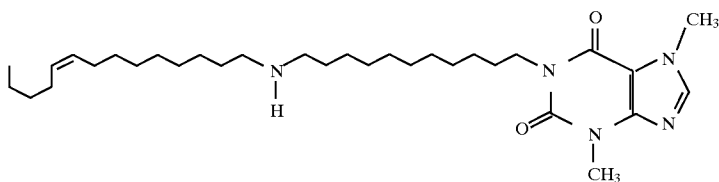
6570 1-[11-(cis-9-Tetradecenylamino)undecyl]-3,7-dimethylxanthine
