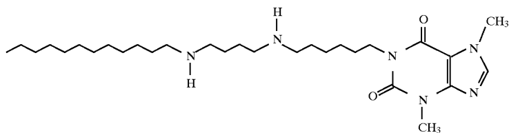
6560 1-(6-[4-Dodecylaminobutylamino]hexyl)-3,7-dimethylxanthine
