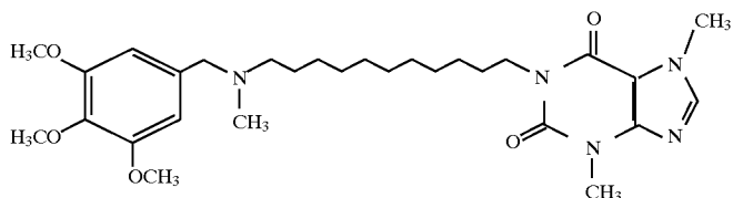
6571 1-[11-(N-Methyl-N-[3,4,5-trimethoxybenzyl]amino)undecyl]-3,7-dimethylxanthine
