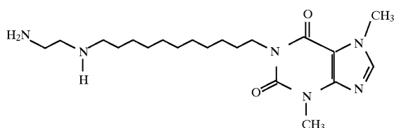
6504 1-[11-(2-aminoethyl)amino]undecyl]-3,7-dimethylxanthine
