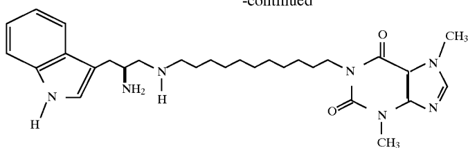
6515 1-[11-(2-amino-3-indolylpropylamino)undecyl]-3,7-dimethylxanthine
