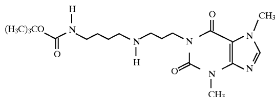
6533 1-(3-[4-Carbobutoxyaminobutylamino]propyl)-3,7-dimethylxanthine
