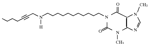
7510 1-[11-[(2-Heptyn-1-yl)amino]undecyl]-3,7-dimethylxanthine
