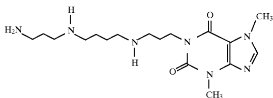
6553 1-(3-[4-(3-Aminopropylamino)butylamino]propyl)-3,7-dimethylxanthine
