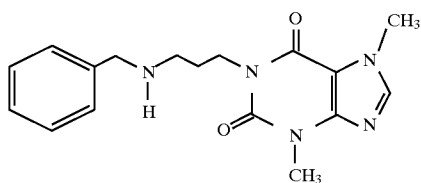
6503 1-(3-Benzylaminopropyl)-3,7-dimethylxanthine
