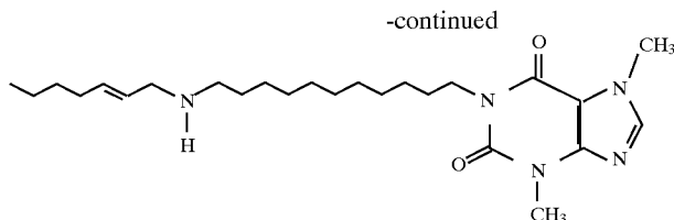
7511 1-[11-[(2-trans-Hepten-1-yl)amino]undecyl]-3,7-dimethylxanthine
