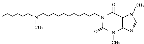
4500 1-[11-(N-Methyl-N-hexylamino)undecyl]-3,7-dimethylxanthine
