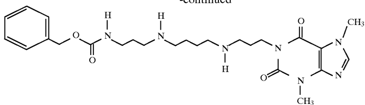
6552 1-(3-[4-(3-Carbobenzyloxyaminopropylamino)butylamino]propyl)-3,7-dimethylxanthine
