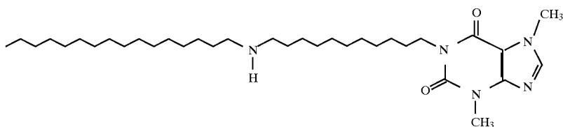
3584 1-(11-Hexadecylamioundecyl)-3,7-dimethylxanthine
