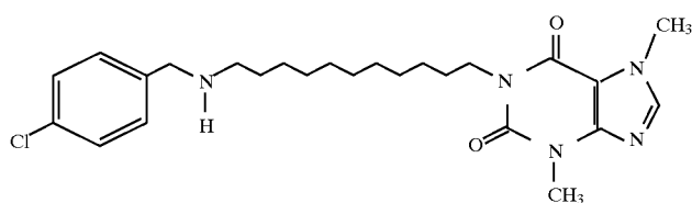
4569 1-(11-(4-Chlorobenzylamino)undecyl)-3,7-dimethylxanthine
