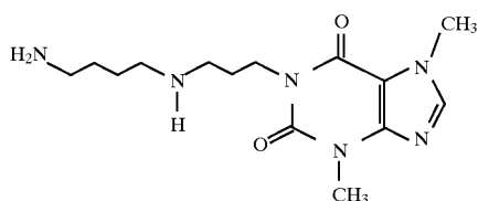
6532 1-(3-[4-Aminobutylamino]propyl)-3,7-dimethylxanthine
