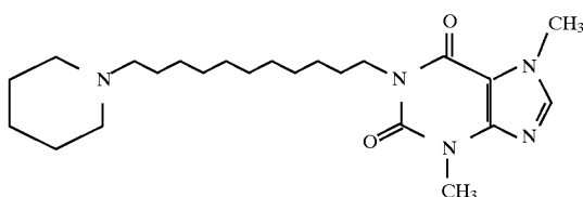
6543 1-[11-(Piperidiny)undecyl]-3,7-dimethylxanthine
