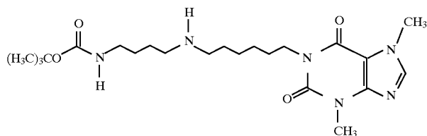
6558 1-(6-[4-(3-Tert-butoxyaminobutylamino)hexyl]-3,7-dimethylxanthine
