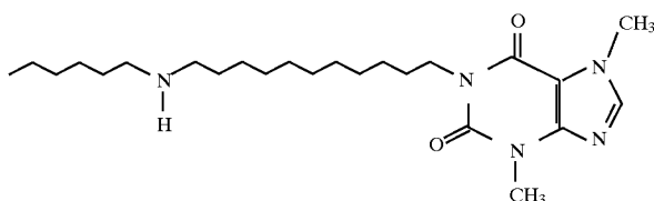
3580 1-(11-Hexylaminoundecyl)-3,7-dimethylxanthine
