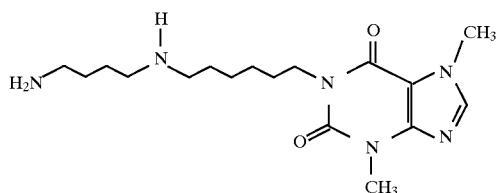
6559 1-(6-[4-(3-Aminobutylamino)hexyl]-3,7-dimethylxanthine
