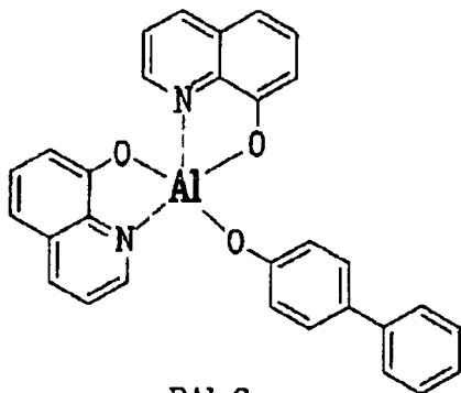
BAlq3
