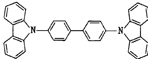
CBP
