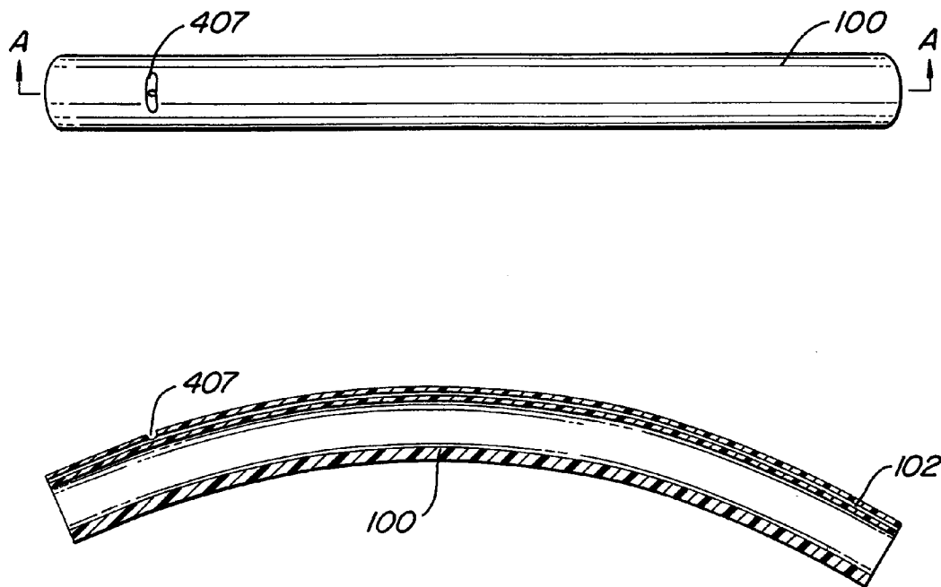
Section A-A FIG. 9
