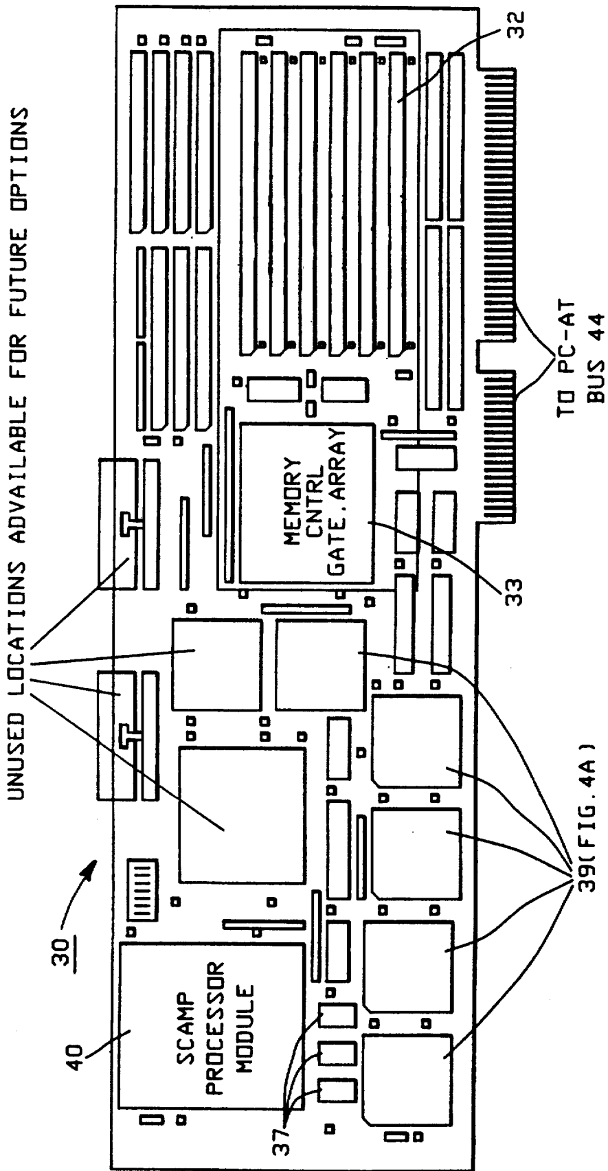
FIG. 4B
