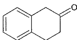
2-tetralone
