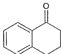
1-tetralone
