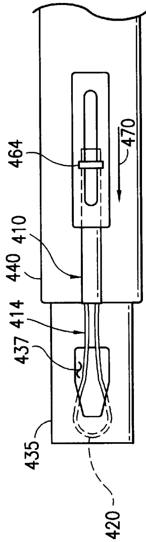
FIG. 30b
