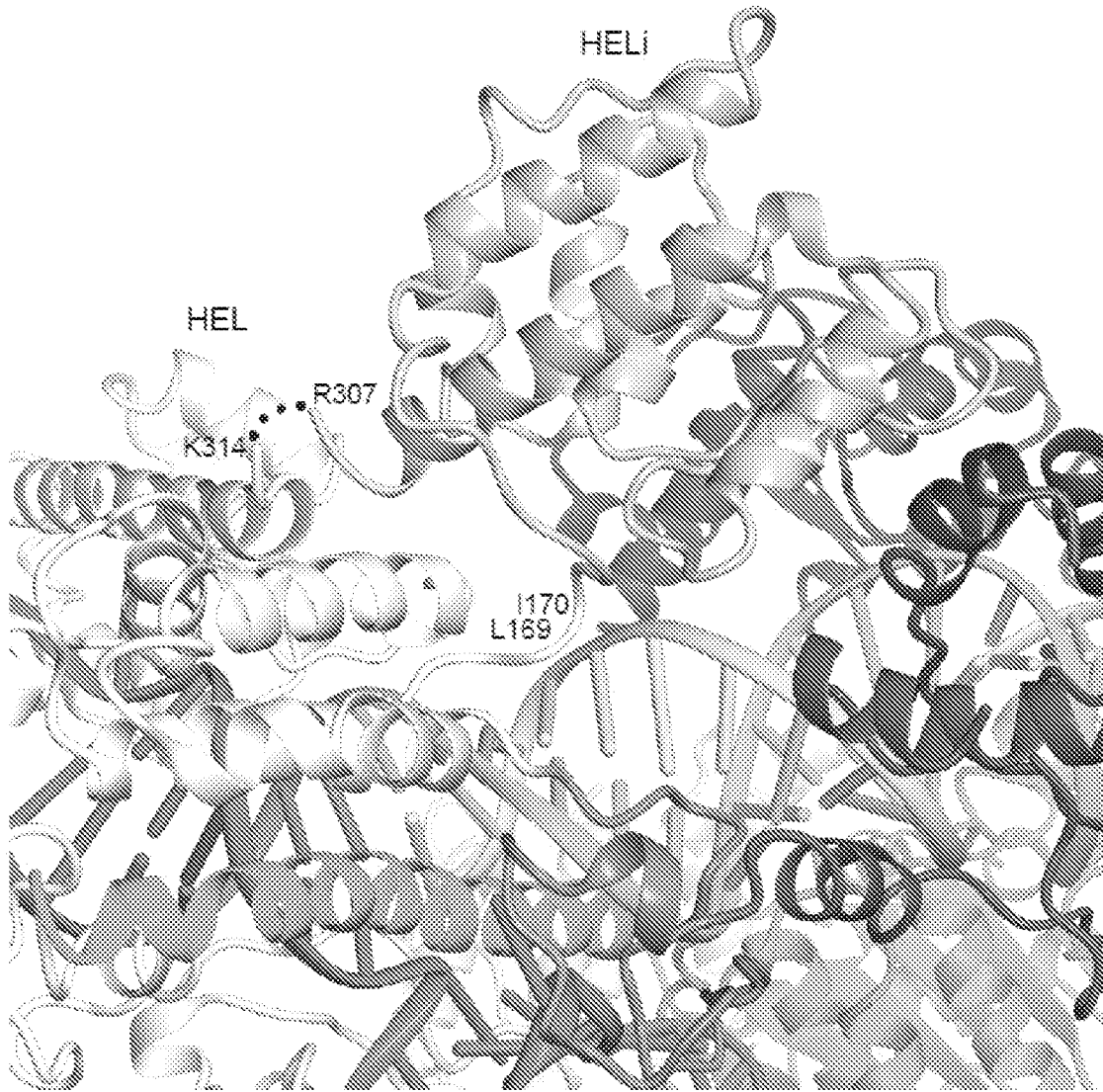
HEL (L169)-linker-Effector-linker-HEL (K314)
