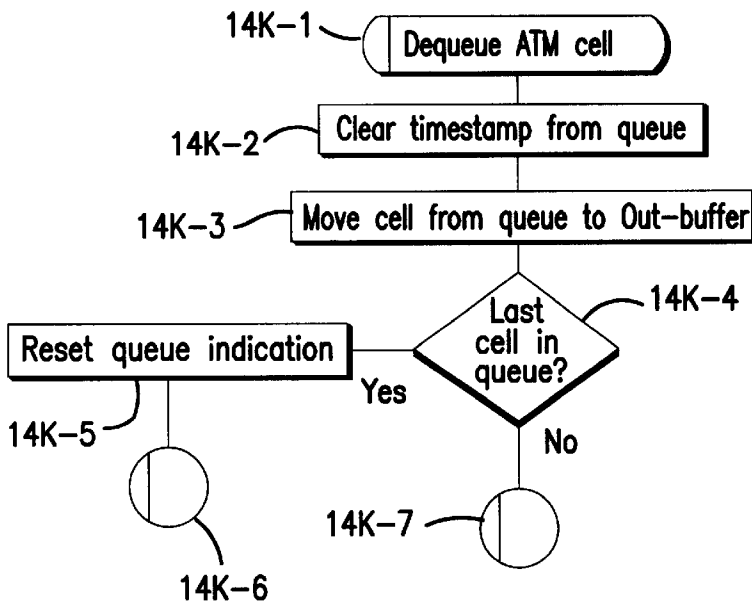
FIG. 14K DEQUEUE ATM CELL FUNCTION
