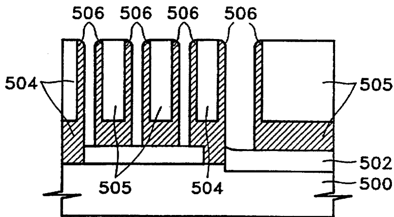
FIG. 1B(PRIOR ART)
