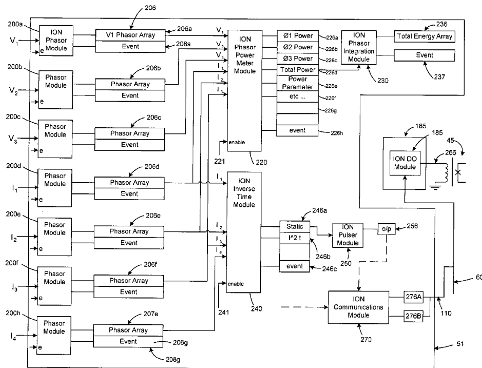
Phasor ION Module Diagram
