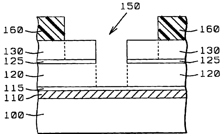
FIG. 1e - Prior Art
