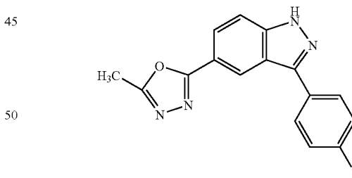
3-(4-Fluoro-phenyl)-5-(5-methyl-[1,3,4]oxadiazol-2-yl)-1H-indazole
