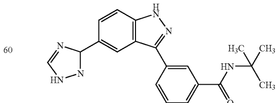
N-tert-Butyl-3-[5-(1H-[1,2,4]triazol-3-yl)-1H-indazol-3-yl]-benzamide
