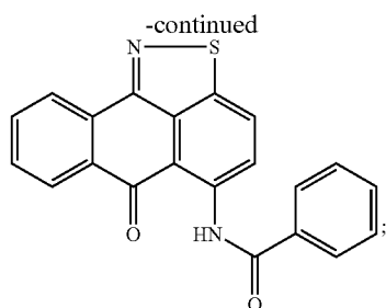
N-(6-Oxo-6H-anthra[9,1-cd]isothiazol-5-yl)-benzamide
