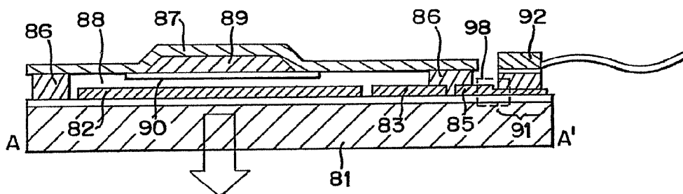
FIG.20C
