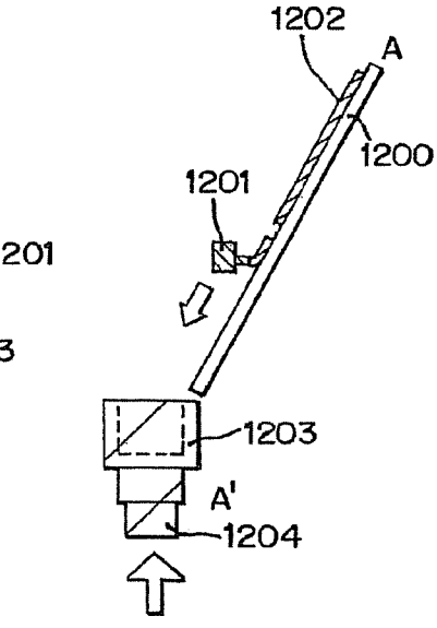
FIG.12B
