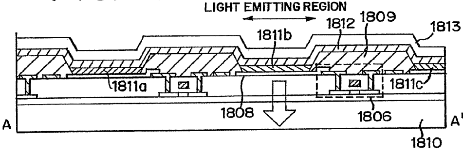
FIG.18B
