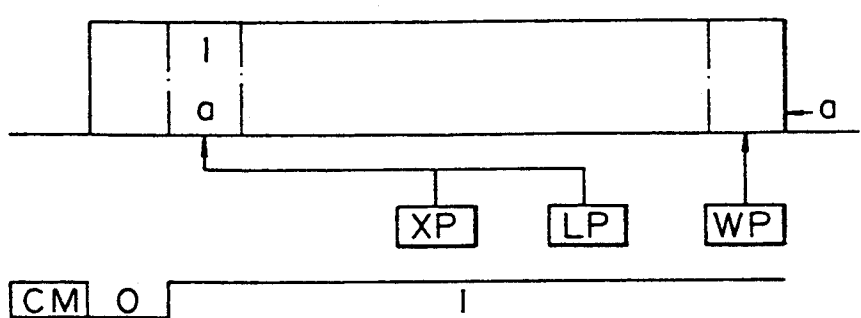
Fig. 14B (ADD)
