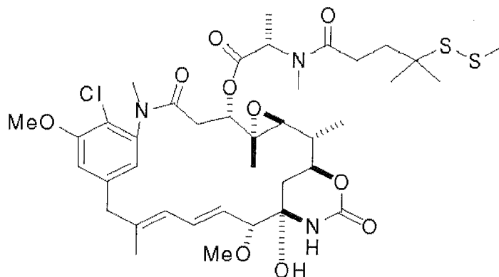
L-DM4-SMe
