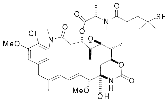
L-DM4
