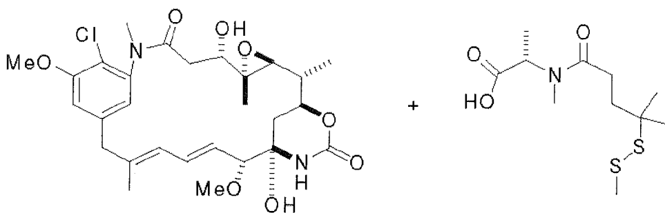
Maytansinol
