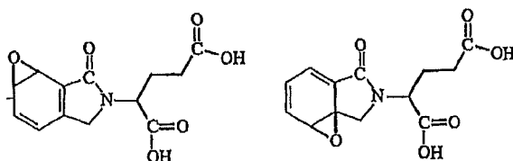
Epoxides of EM 138
