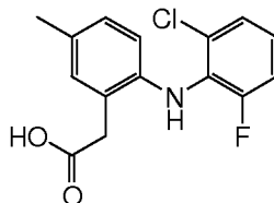
Lumiracoxib
