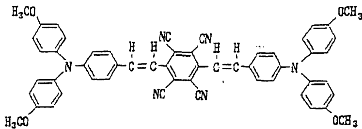
Strukturformel (3)-4:
