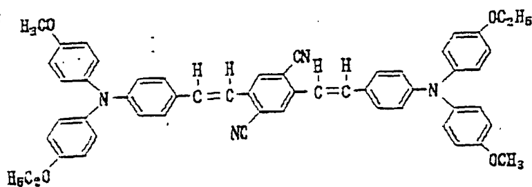
Strukturformel (3)-2:
