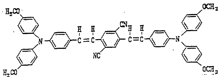
Strukturformel (3)-1:
