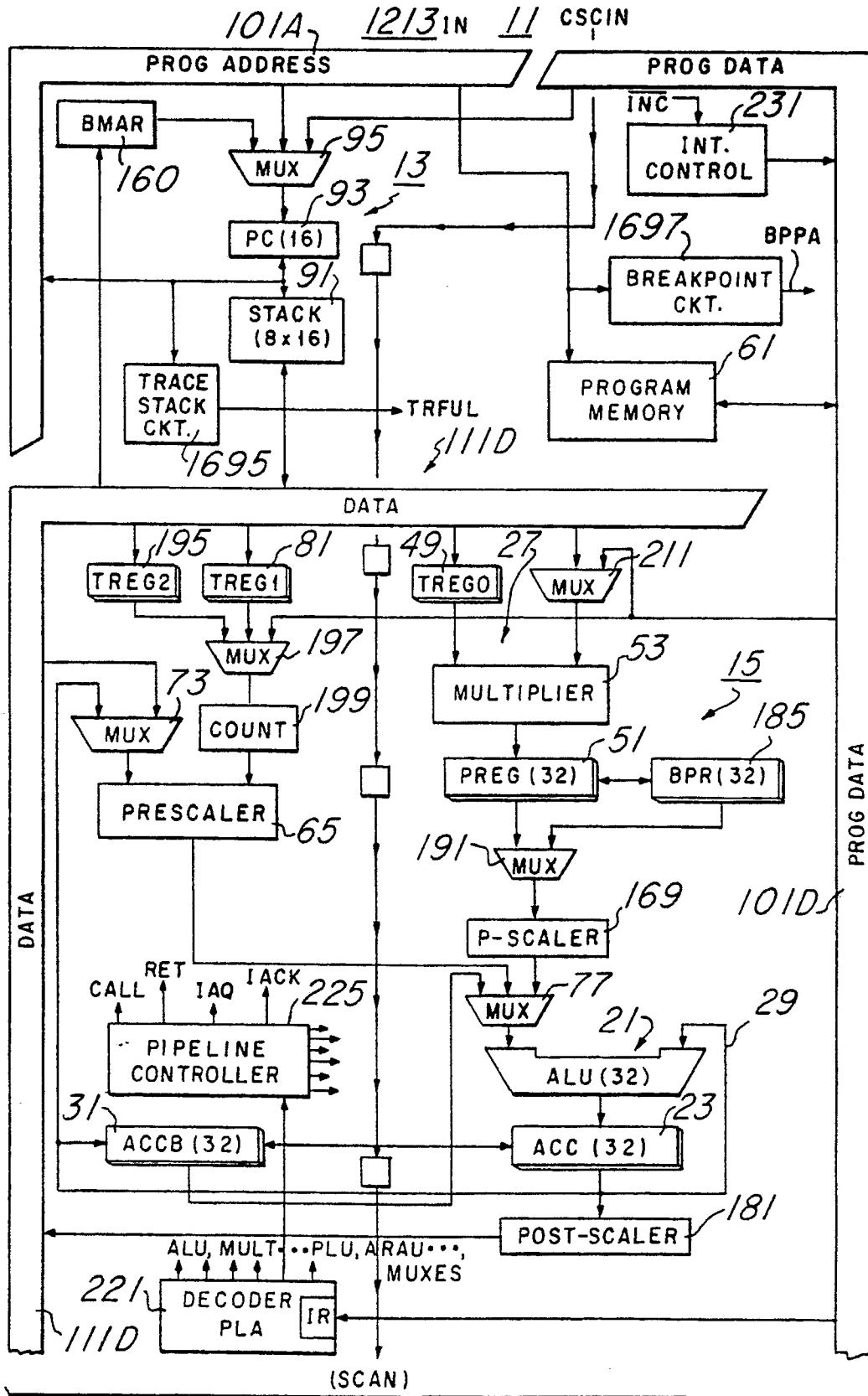
FIG. 25A JOIN FIG.68B
