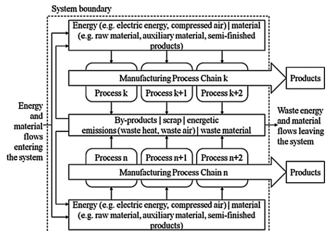
Fig. 12. Multi-machine ecosystem.
