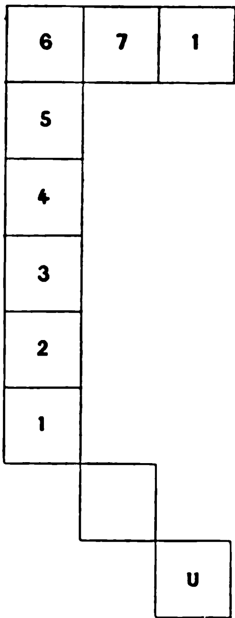
Théorème de l'angle droit.
